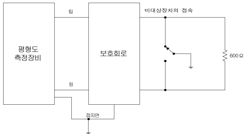
(그림 2) 유선분야의 적합성평가 대상이 아닌 기기를 접속하기 위한 종단회로(2선식)
